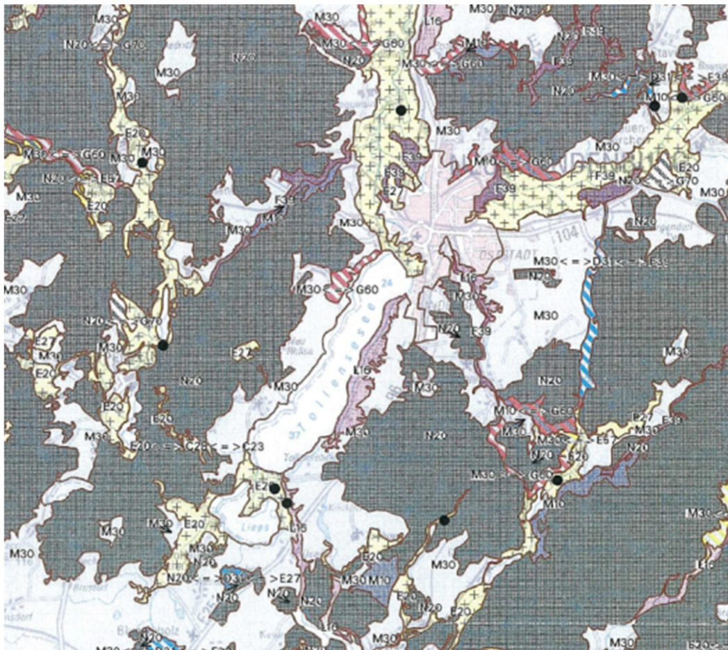
Bild 3: Übersicht der HPNV-Einheiten
