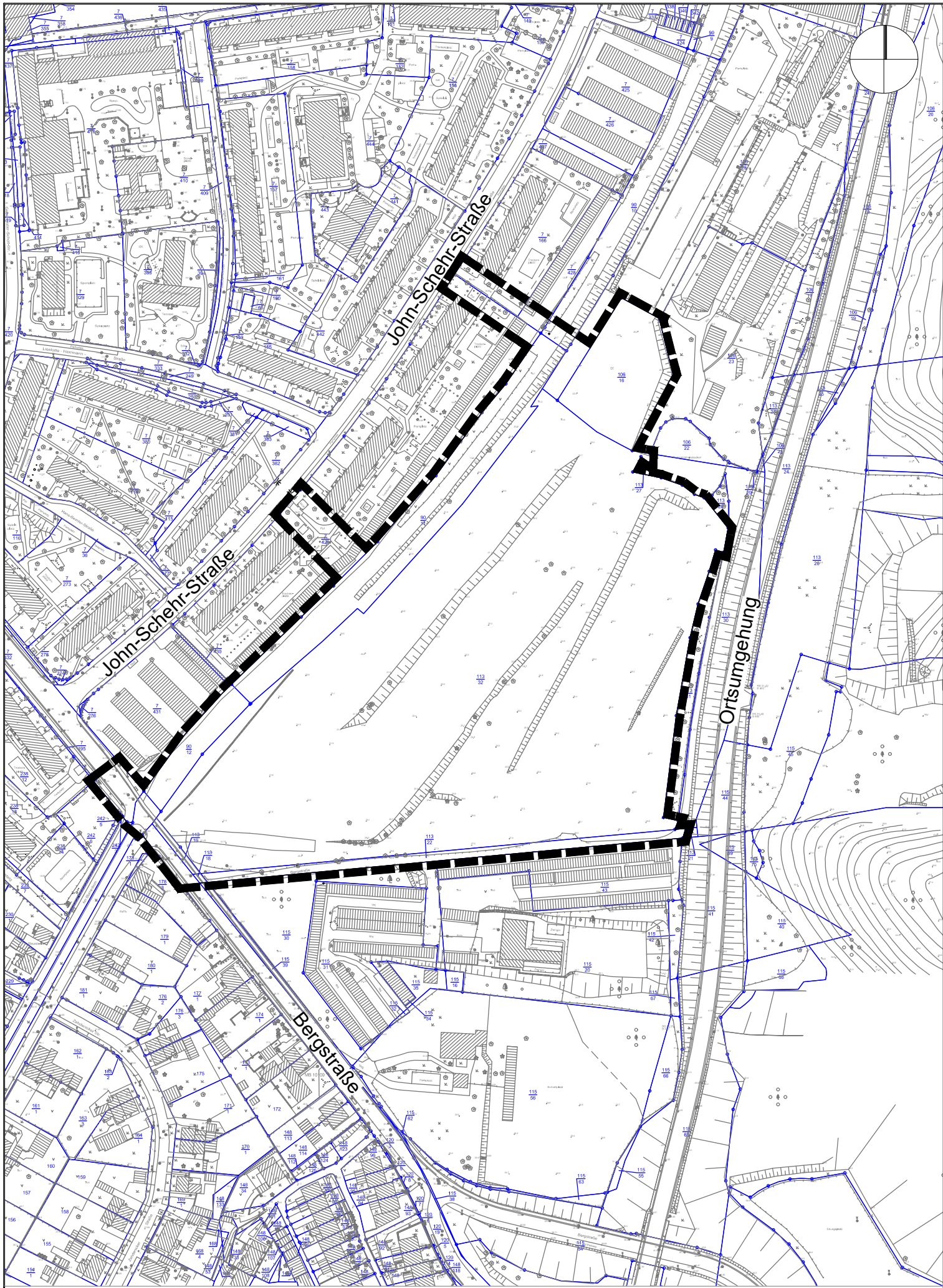
█ Geltungsbereich des Bebauungsplanes Nr. 45 "Ehemaliges Betonwerk Süd"
